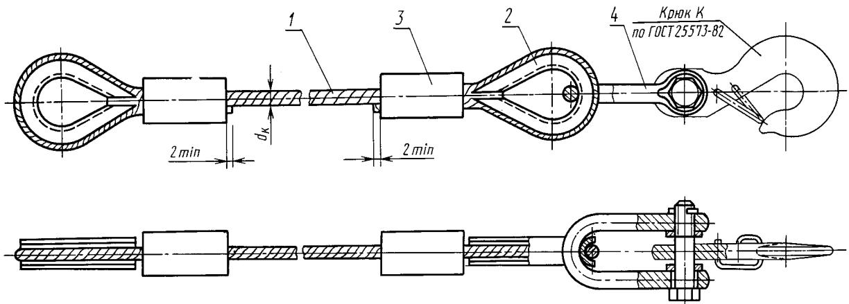
Канатная ветвь с переходным звеном
